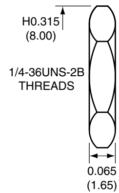
NUT
